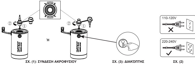
ΣΧ. (1): ΣΥΝΔΕΣΗ ΑΚΡΟΦΥΣΙΟΥ
